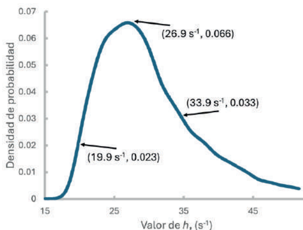
Figura 10. Resultados Montecarlo de la estimación de la constante de enfriamiento.
