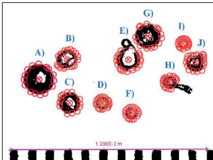
Figura 7. Imagen de las muestras etiquetadas para cada partícula y los puntos marcados para ajustar circunferencias para calcular el radio.
