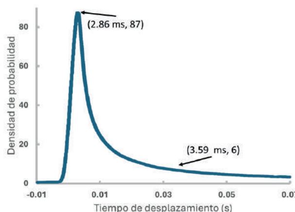
Figura 9. Resultados Montecarlo de la estimación del tiempo de fundición del glóbulo de cobre.
