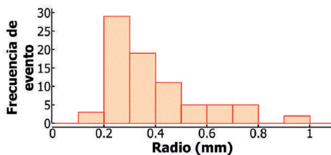
Figura 8. Distribución de los radios de las partículas producidas durante las pruebas de cortocircuito.
