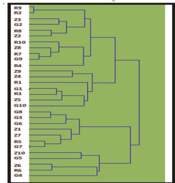
Gráfica 1. Dendrograma
