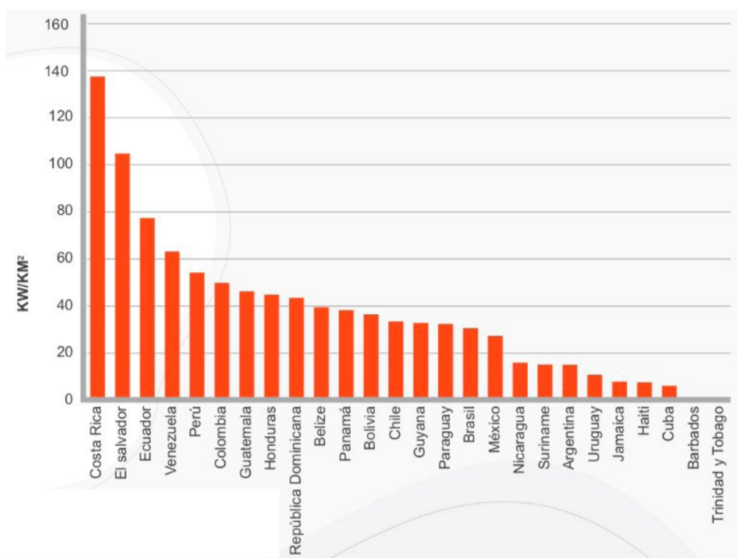
Densidad de potencial hidroeléctrico para Latinoamérica
